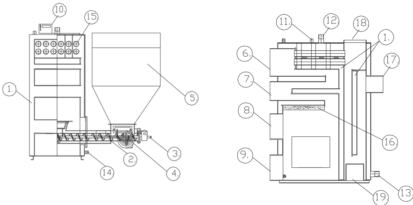
Rysunek 1. Kocioł Klaster 5-75 o mocy 75 kW z palnikiem retortowym – widok ogólny.
