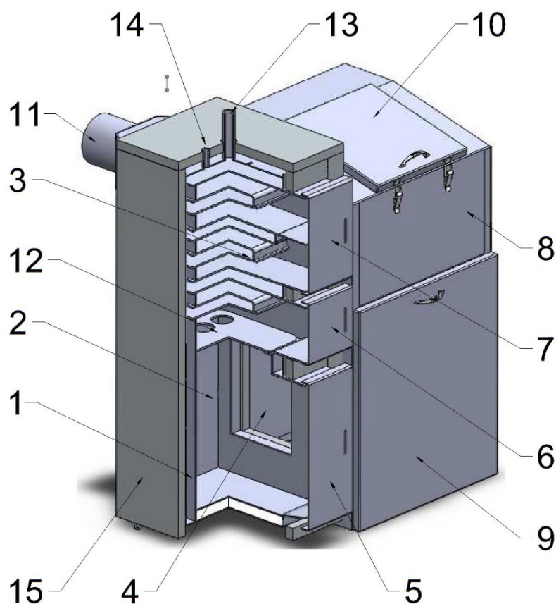
Rys.1. Kocioł „Technix Eco-Premium”
