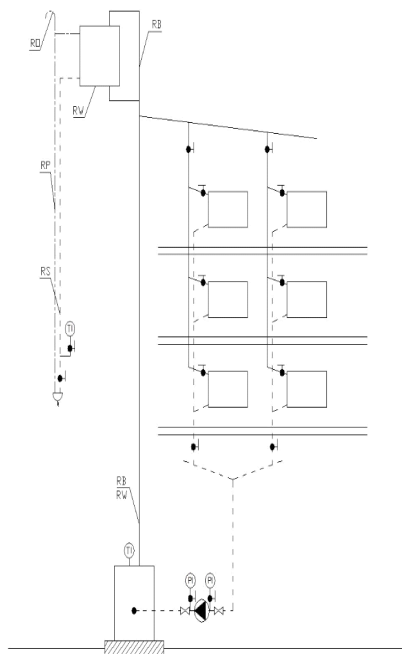
Rysunek 1b Schemat zabezpieczenia instalacji ogrzewania wodnego, wyposażonej w jeden kocioł lub wymiennik ciepła, rozdziel górny, pompa zamontowana na powrocie wg PN-91/B-02413
