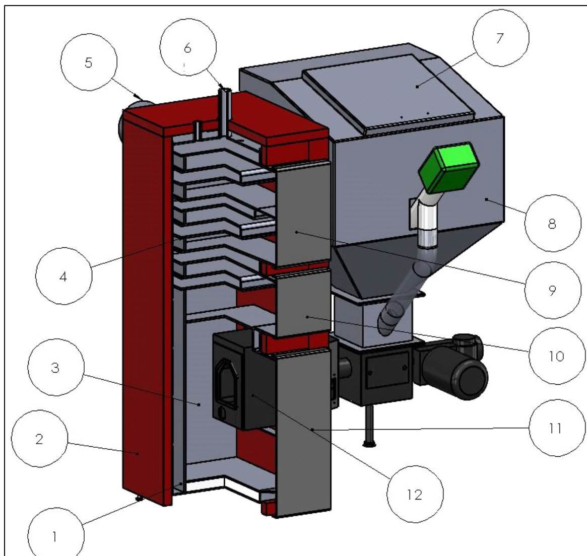
Rys.1. Kocioł "Technix-Pel"
