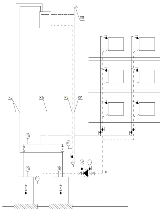
Rysunek 1c Schemat zabezpieczenia instalacji ogrzewania wodnego, wyposażonej w dwa lub więcej kotły lub wymienniki ciepła, rozdziel górny, pompa zamontowana na powrocie wg PN-91/B-02413
